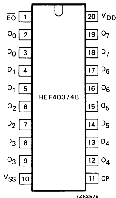
Fig.2 Pinning diagram.
